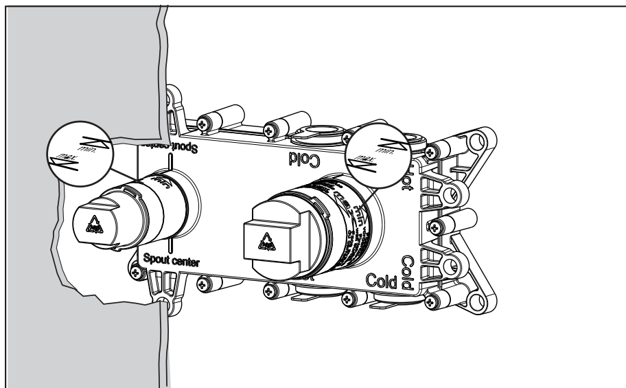
MONTAGGIO SU PARETE IN CARTONGESSO MOUNTING ON PLASTERBOARD WALL
